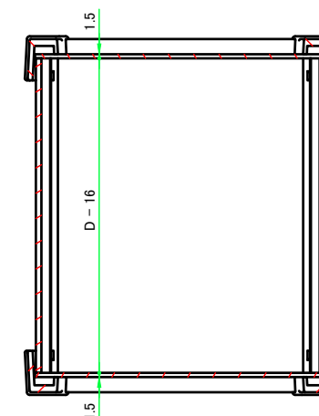
C-C ( 1 : 2.5 )
