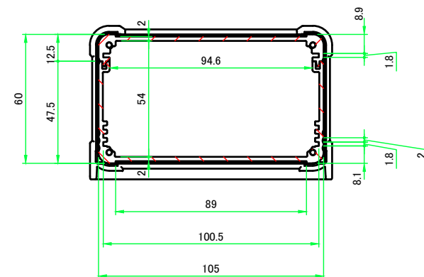
A-A ( 1 : 2.5 )
